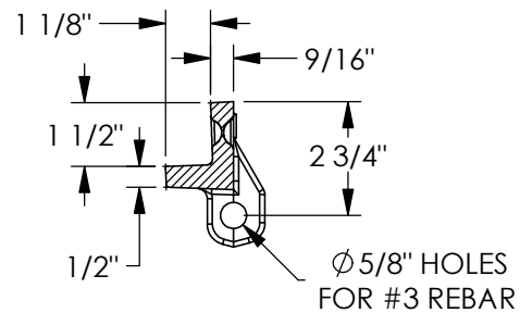
SECTION A-A SCALE 1 : 5
