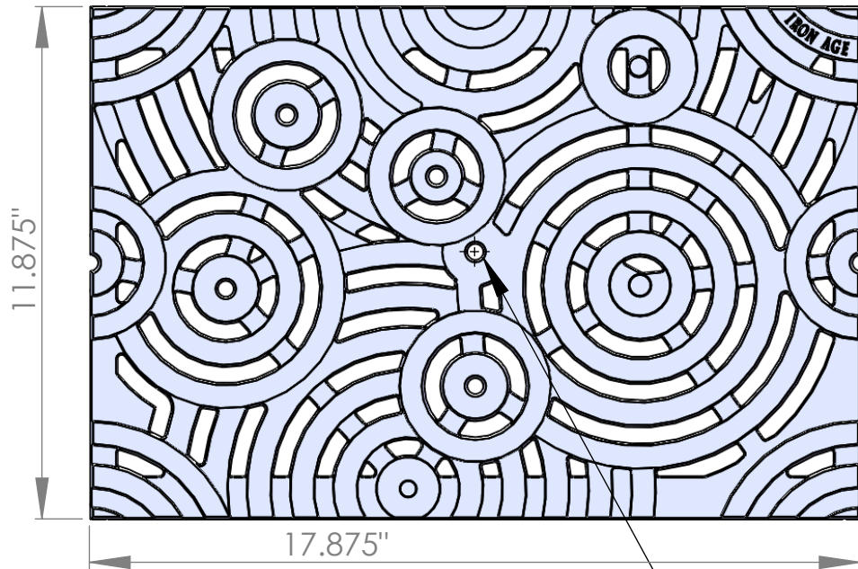
TOP scale 1:4
